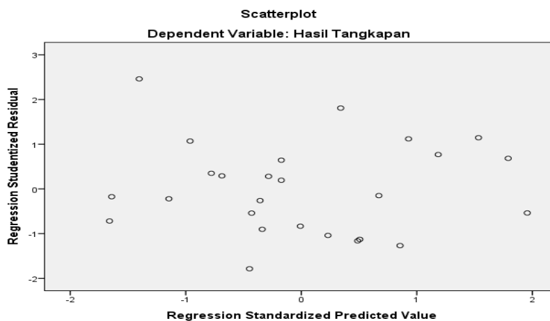
Gambar 4. Scatterplot hasil pengelolaan SPSS
