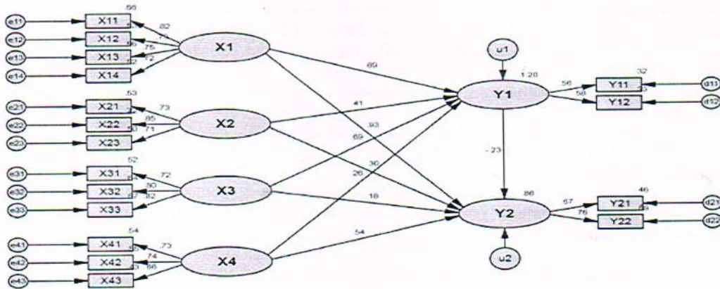
matriks dan estimasi model
