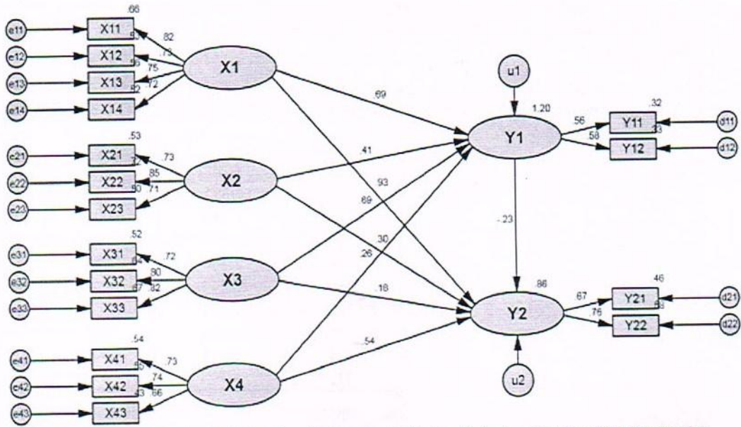
Matriks dan estimasi Model Struktur hubungan Indikator Terhadap Variabel (X1,X2,X3,X4)
