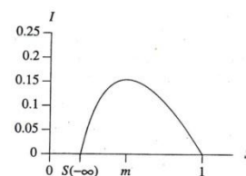
Gambar 3. Bidang fase (S, I)
