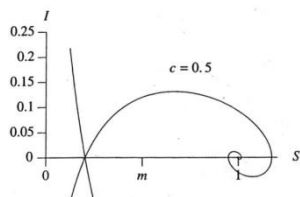
Gambar 4. Fokus stabil untuk c < 2\sqrt{1 - m}
