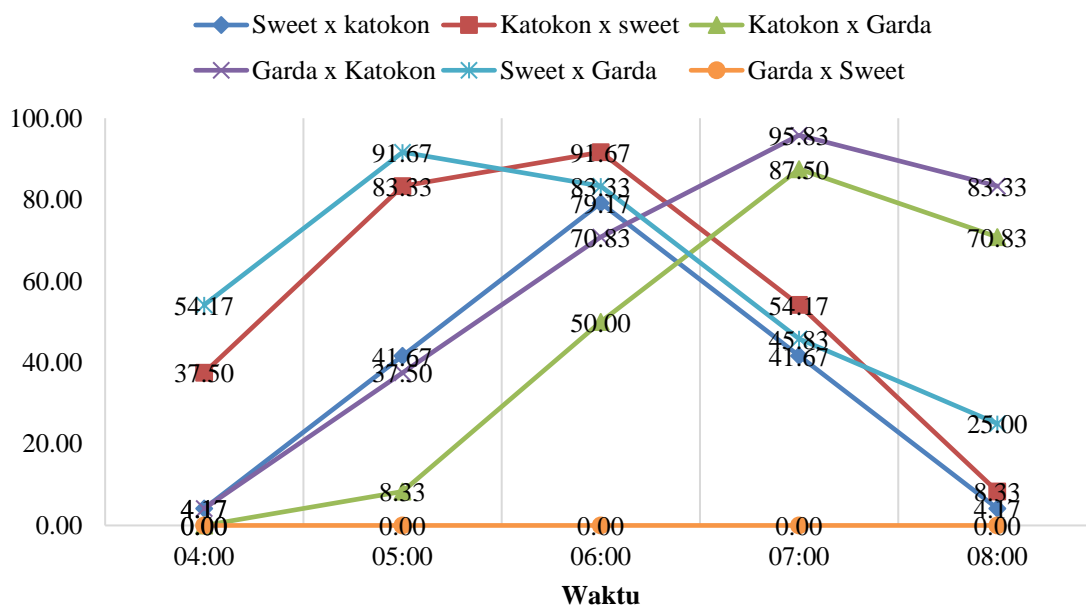
Gambar 1. Grafik persentase keberhasilan persilangan
