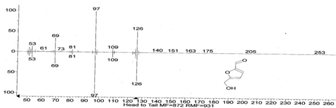
Gambar 3 Spektrogram fraksinasi massa senyawa puncak 5
