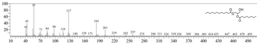
Gambar 11. Spektrum MS 2-laurin, 3-kaprolin diasilgliserol
