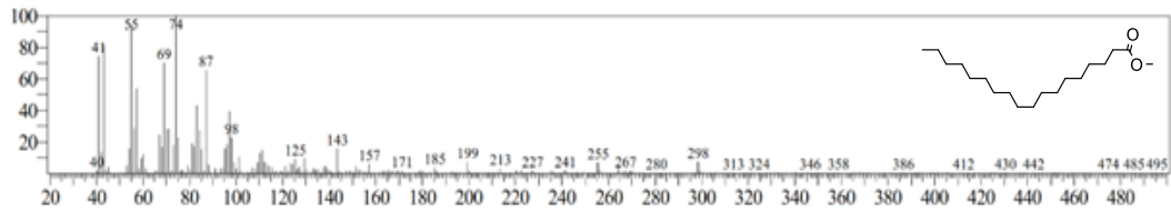
Gambar 5. Spektrum MS metil ester stearat
