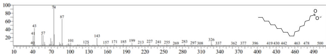
Gambar 7. Spektrum MS metil ester arachidat
