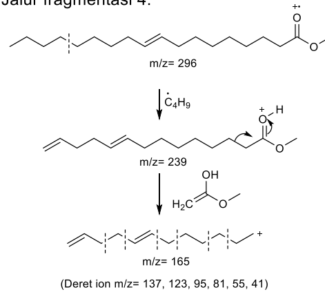
Gambar 4. Mekanisme fragmentasi metil ester oleat
