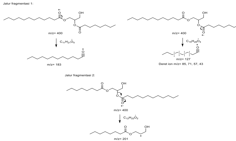
Gambar 12. Mekanisme fragmentasi 2-laurin, 3-kaprolin diasilgliserol
