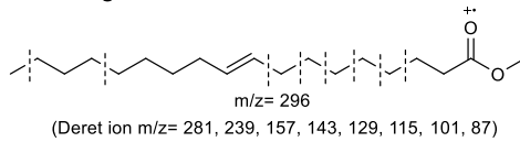
Gambar 4. Mekanisme fragmentasi metil ester oleat
