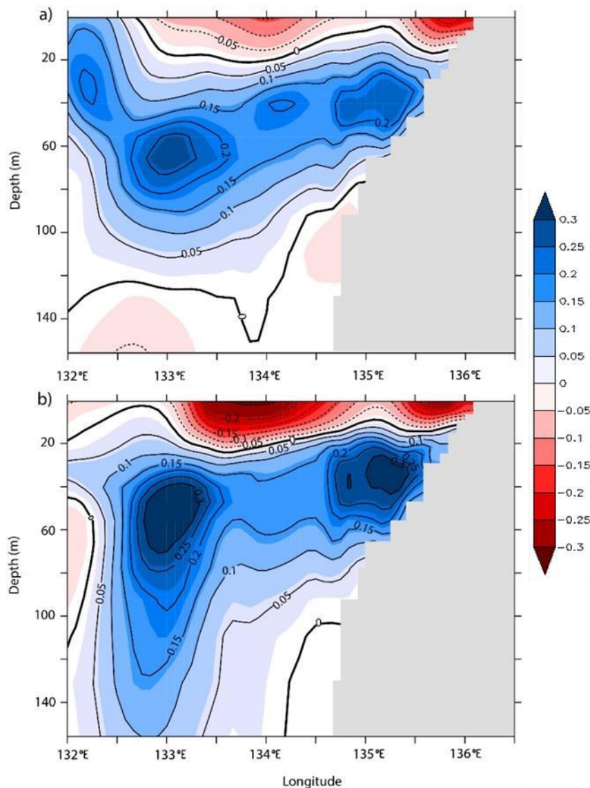
Gambar 5. Penampang melintang rerata arus komponen timur-barat (zonal) selama periode monsoon tenggara (Juni-September) pada koordinat 4.6°LS dan 132°BT - 136.5°BT sepanjang tahun kejadian super ENSO. a) La Nina (2010); b) El Nino (2015). Nilai dan warna pada skala-bar menunjukkan kecepatan (m/s) dan arah. Nilai positif (warna biru) menunjukkan arus ke arah timur (menuju pantai), sedangkan nilai negatif (warna merah) menunjukkan arus ke arah barat (meninggalkan pantai).
