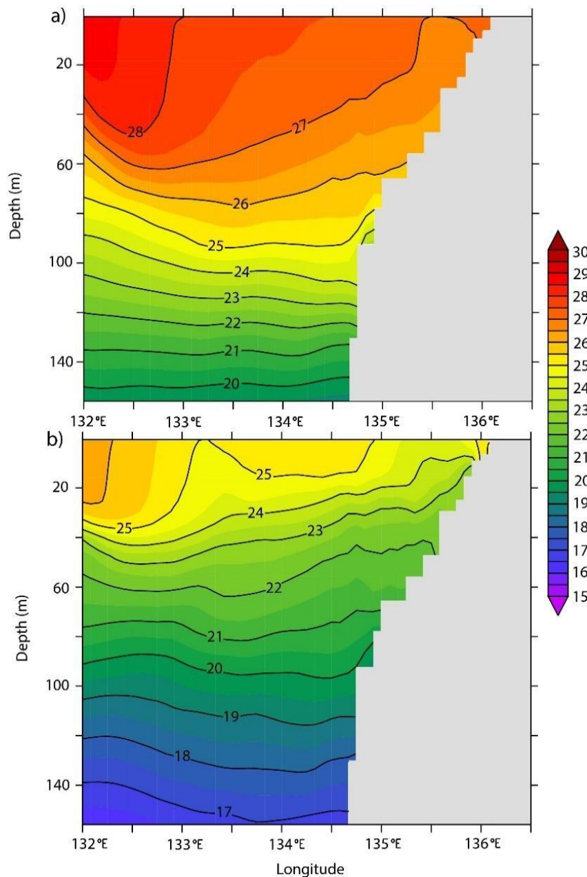
Gambar 4. Penampang melintang rerata suhu selama periode angin Monsun Tenggara (Mei-September) pada koordinat 4.6°LS dan 132°BT – 136.5°BT sepanjang tahun kejadian super ENSO. a) La Nina (2010); b) El Nino (2015).
