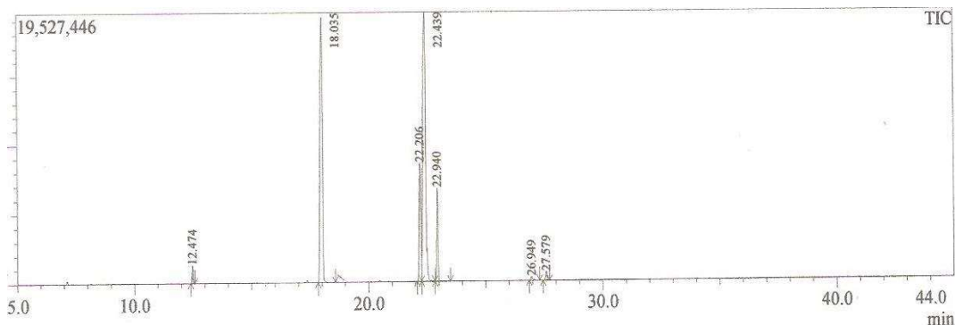
Gambar 5. Kromatogram metil ester (biodiesel).
