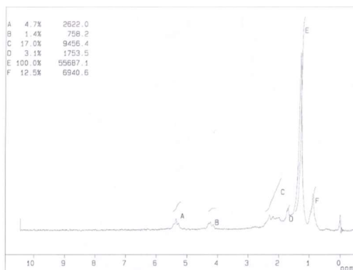
Gambar 3. Spektra 1 H-NMR minyak goreng bekas
