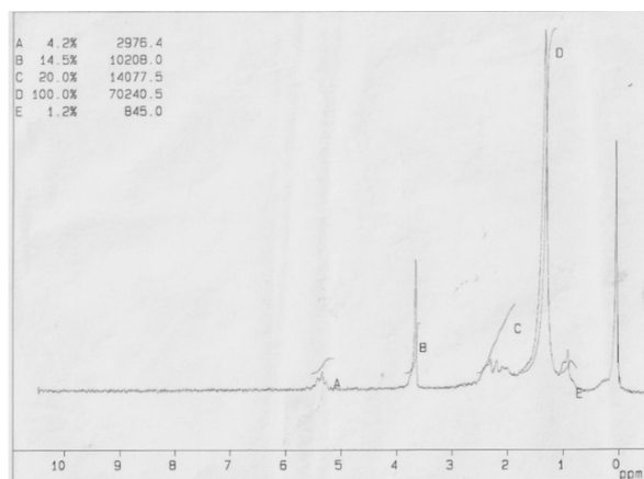
Gambar 4. Spektra 1 H-NMR biodiesel
