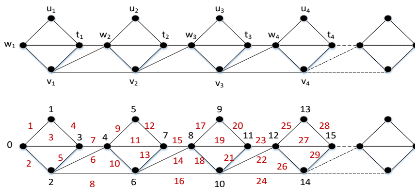
Gambar 2. Konstruksi dan pelabelan graf segitiga belah ketupat LM_n
