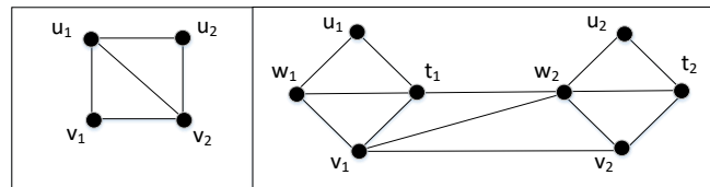
Gambar 1. LS_2 dan LM_2
